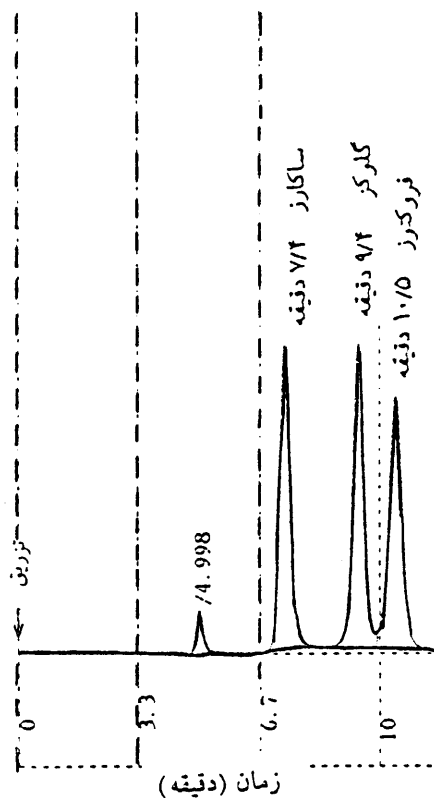
شکل ۲- منحنی نهیبه شده از قندهای موجود در عصاره زیتون کالاماتای تخمیری در روز بیستم تخمیر با دستگاه HPLC در شرایط سیستم ایزوکراتیک، سرعت جریان فاز متحرک ۰/۷ میلی لیتر در دقیقه دمای ستون ۶۰ درجه سانتیگراد با شناسانگر آر-ای-دی
