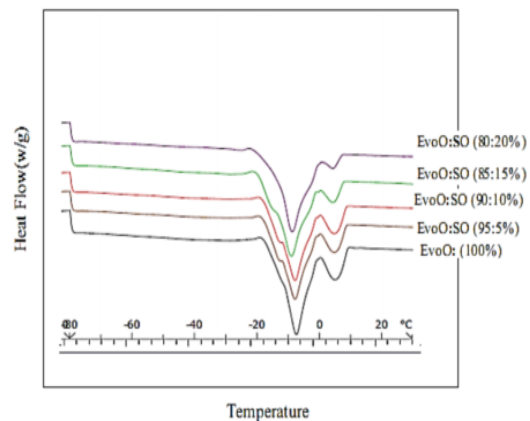
شکل ۲- ترموگرام‌های گرم کردن DSC روغن زیتون فوق بکر و مخلوط ۵، ۱۰، ۱۵ و ۲۰ درصد روغن آفتابگردان با روغن زیتون فوق بکر (EvoO): روغن زیتون فوق بکر و SO: روغن آفتابگردان
