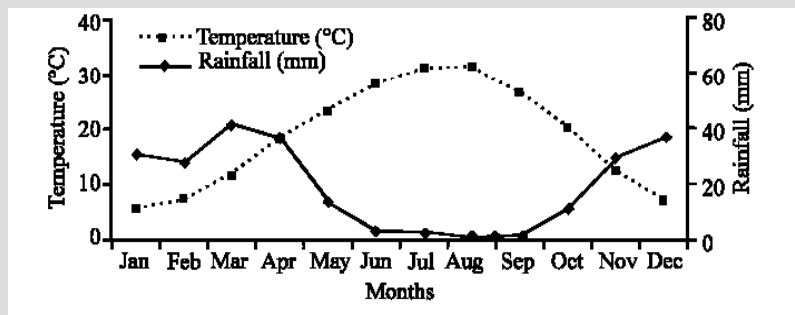
شکل ۱- منحنی آمبروترمیک منطقه مورد مطالعه
